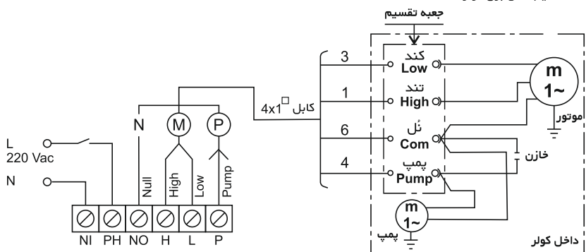
نقشه سیم کشی برق کولر
