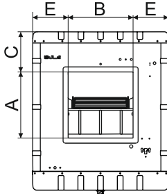
نمای روبرو کولر
